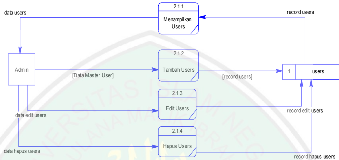
Gambar 3.9 DFD level 3 proses 2.1 manajemen users
