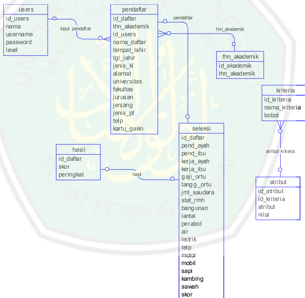
Gambar 3.13 ERD SPK penerima beasiswa
