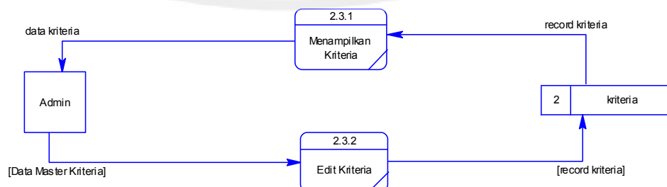
Gambar 3.11 DFD level 3 proses 2.3 manajemen kriteria
