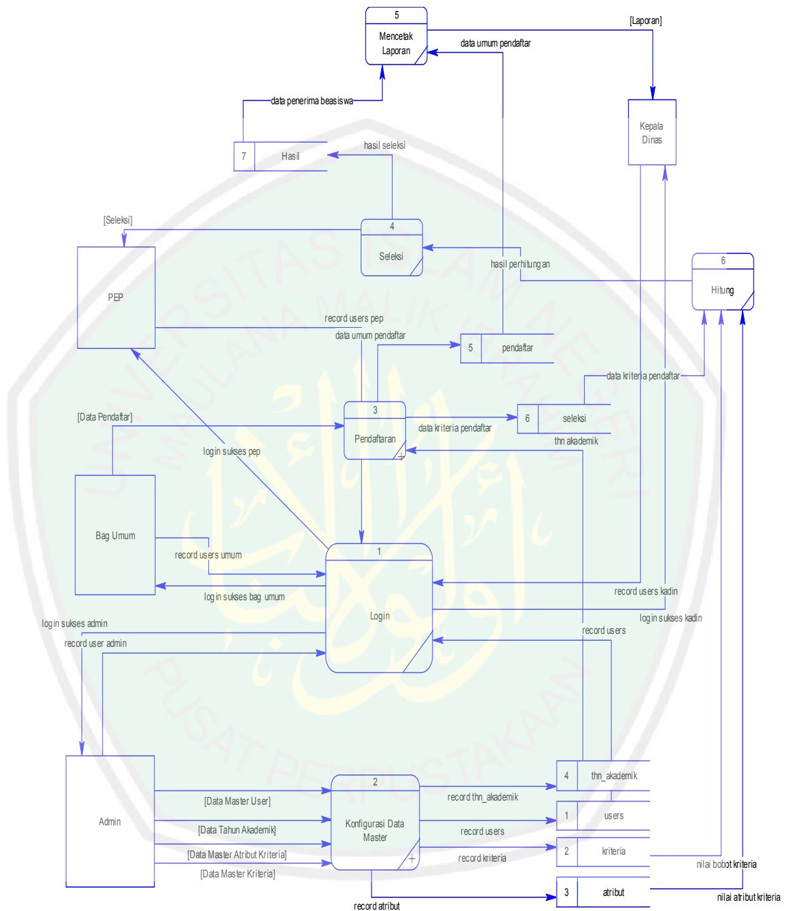
Gambar 3.6 DFD level 1
