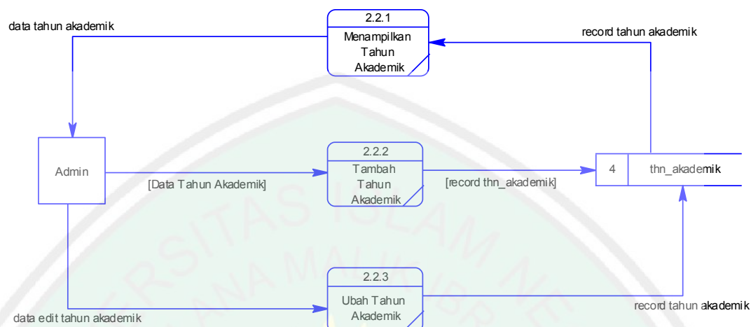
Gambar 3.10 DFD level 3 proses 2.2 manajemen tahun akademik
