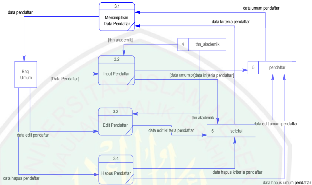
Gambar 3.8 DFD level 2 proses 3 pendaftaran
