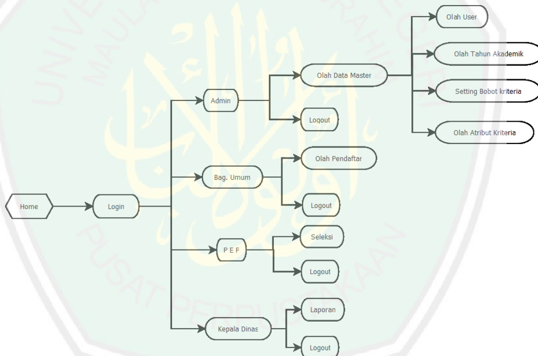
Gambar 3.4 Arsitektur aplikasi
