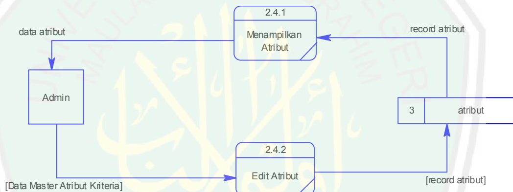
Gambar 3.12 DFD level 3 proses 2.4 manajemen atribut
