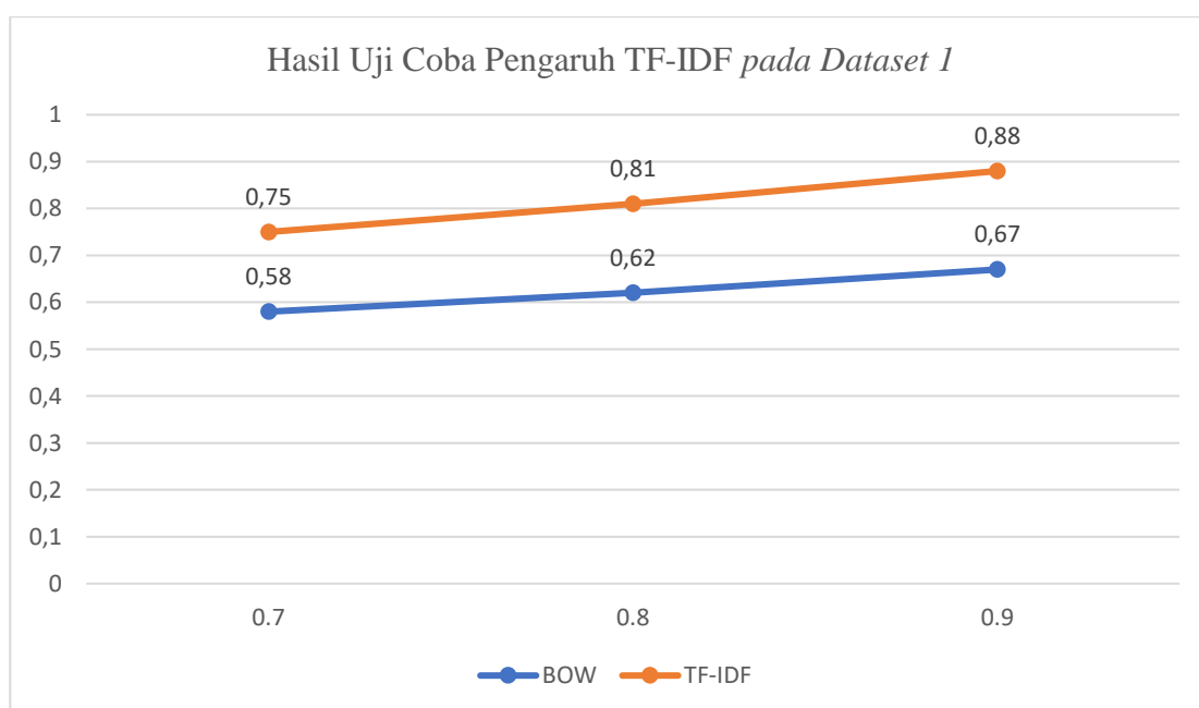
Gambar 4. 1 Grafik Perbandingan Nilai Akurasi pada Dataset 1
