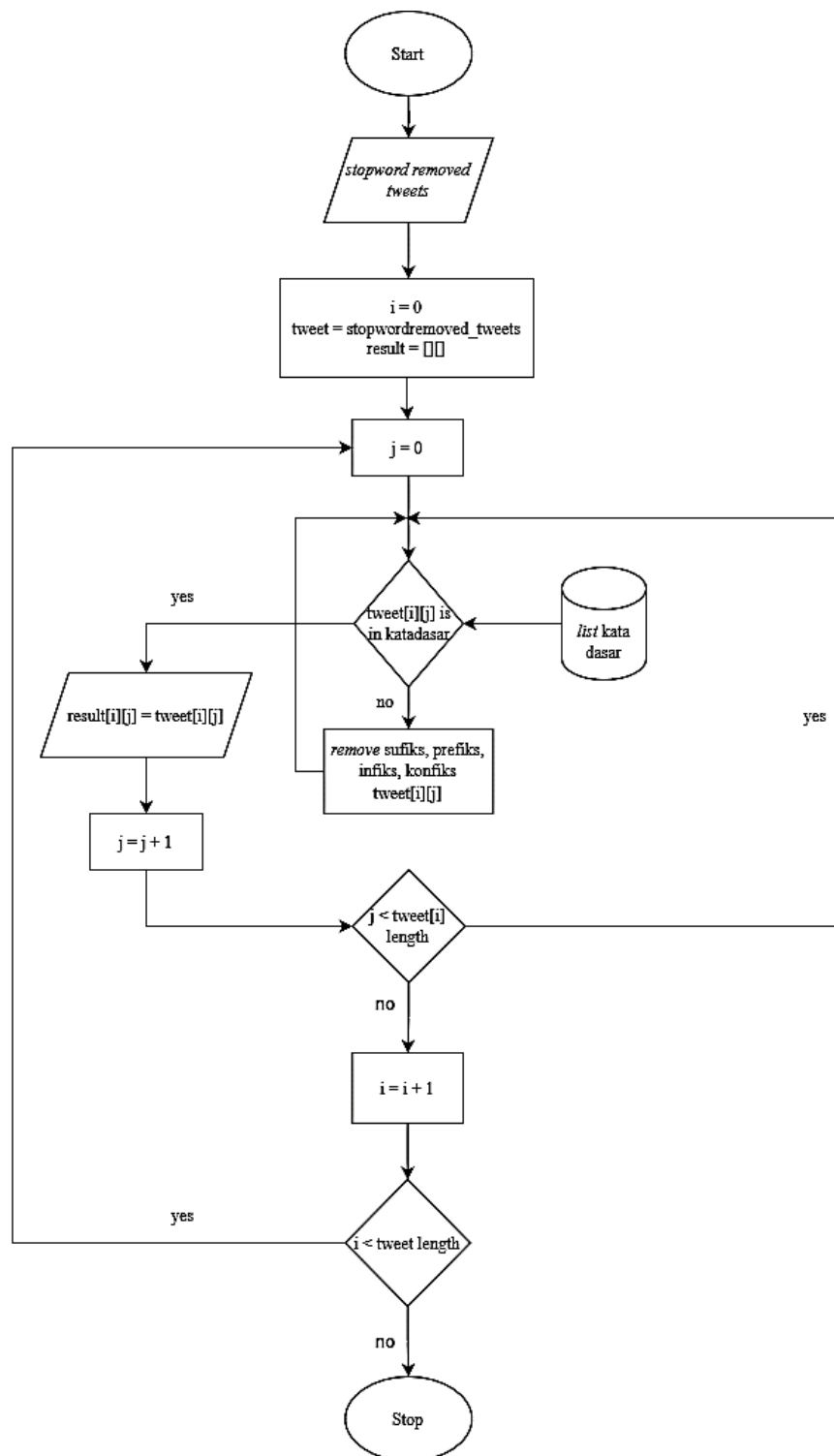
Gambar 3. 5 Flowchart Stemming
