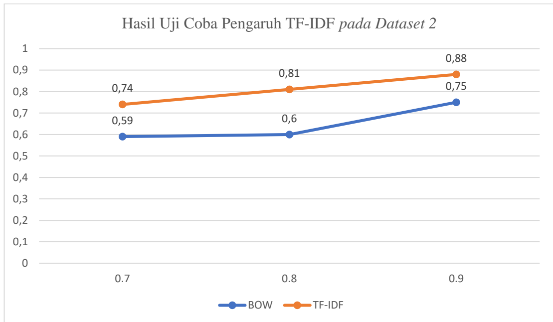
Gambar 4. 2 Grafik Perbandingan Nilai Akurasi pada Dataset 2
