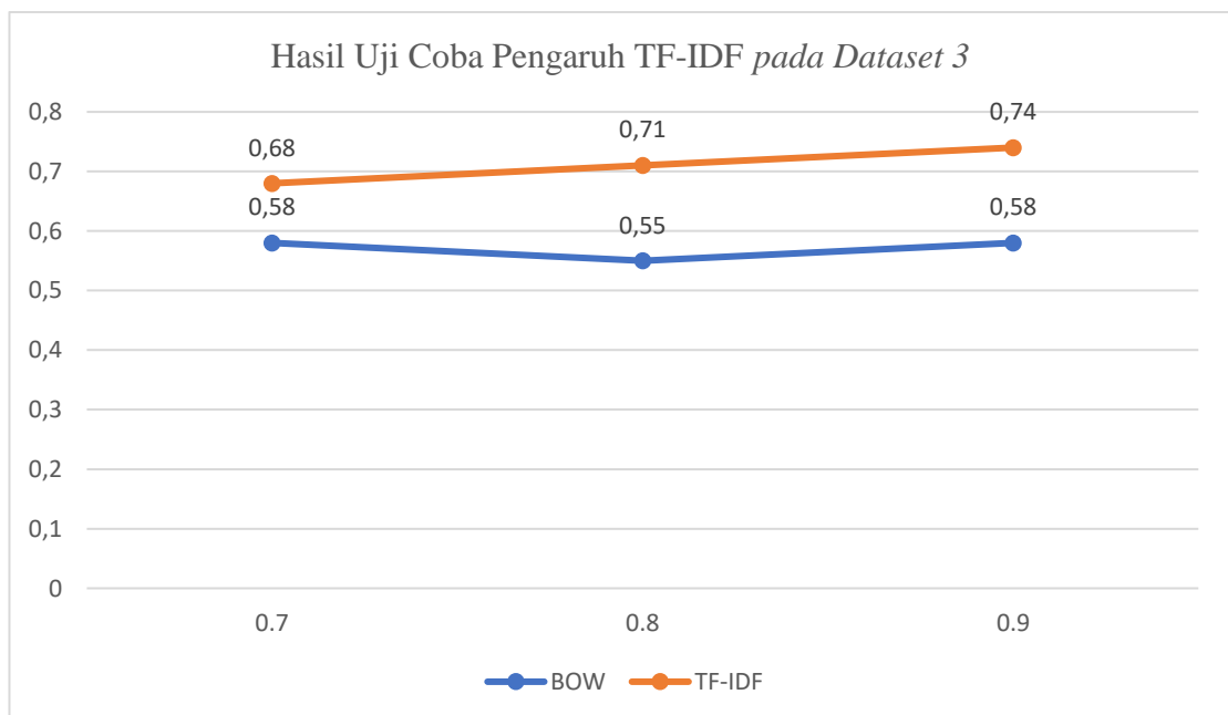
Gambar 4. 3 Grafik Perbandingan Nilai Akurasi pada Dataset 3
