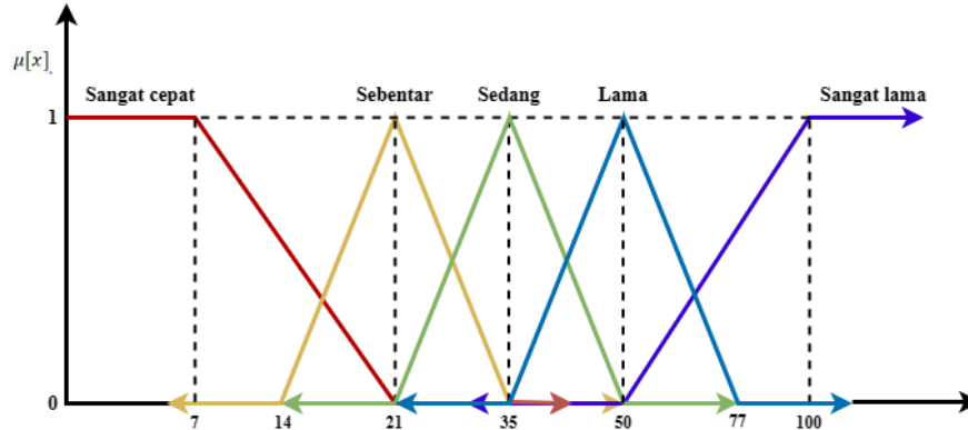
Gambar 4.3. Himpunan Fuzzy Variabel Lama Pengerjaan
