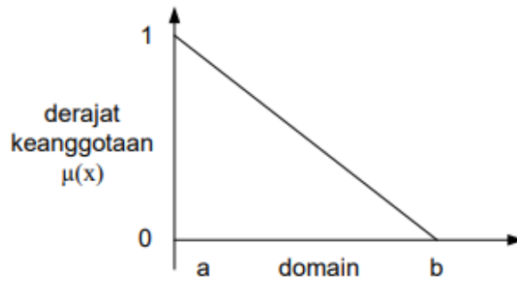
Gambar 2.2. Kurva Linier Turun
