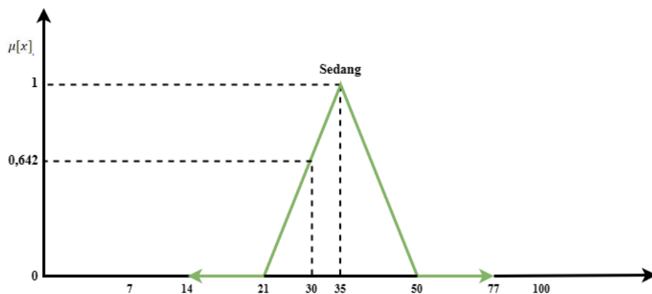
Gambar 4.7. Perhitungan Himpunan Fuzzy Lama Pengerjaan Sedang
