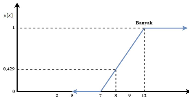
Gambar 4.5. Perhitungan Himpunan Fuzzy Warna Banyak
