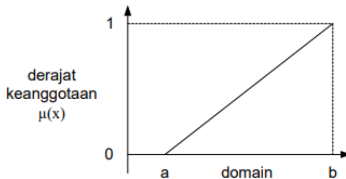
Gambar 2.1. Kurva Linier Naik
