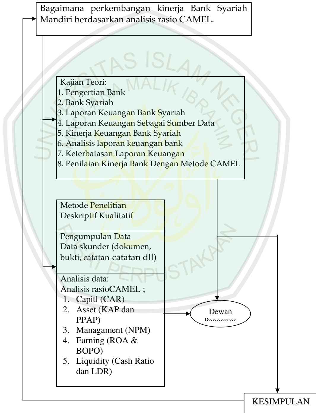
Gambar 2.1 Kerangka Berfikir
