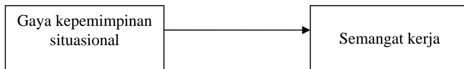
Gambar. 2.3 Model Konsep
