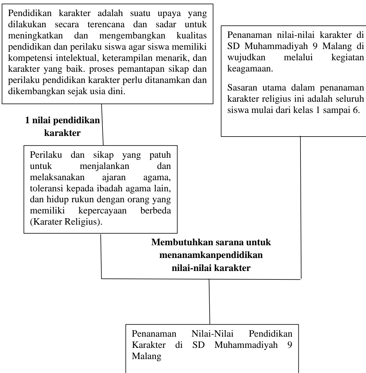
Gambar 2.1 Kerangka Berpikir
