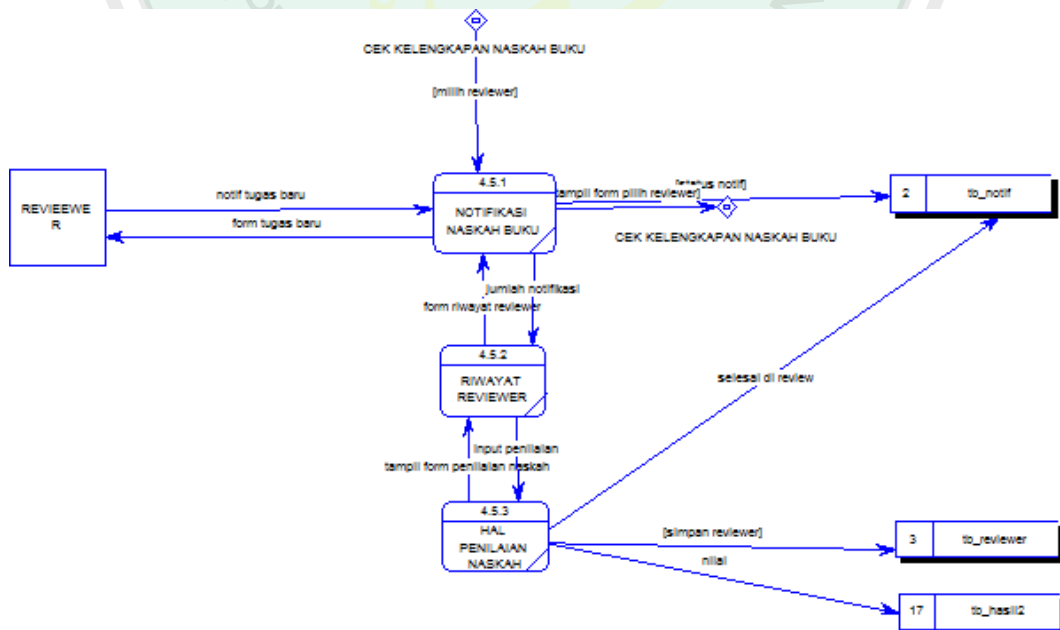
Gambar 3. 22 DFD Level 3 Proses Notifikasi Naskah Baru
