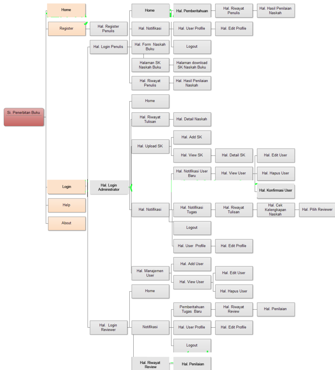
Gambar 3. 16 Sitemap Sistem Penilaian Penerbitan Buku
