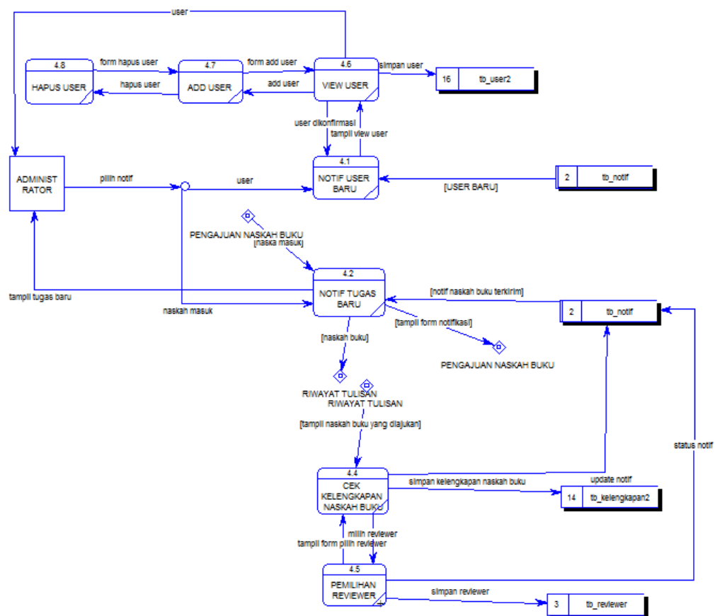
Gambar 3. 21 DFD Level 3 Proses Pemilihan Reviewer
