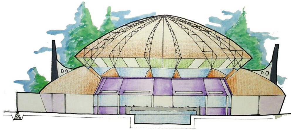
Potongan A-A Aquarium
