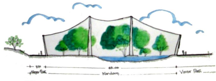
Potongan B-B Kandang Burung Air
