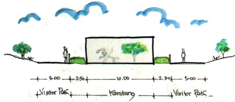
Potongan B-B kandang Ular
