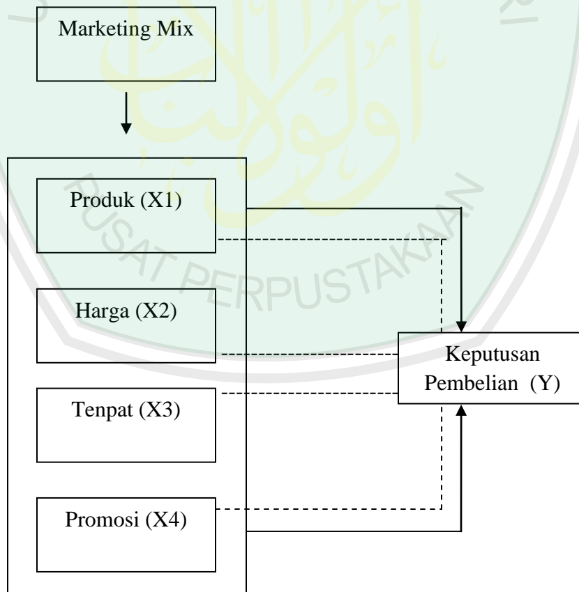
Gambar 2.2 Kerangka Berfikir
