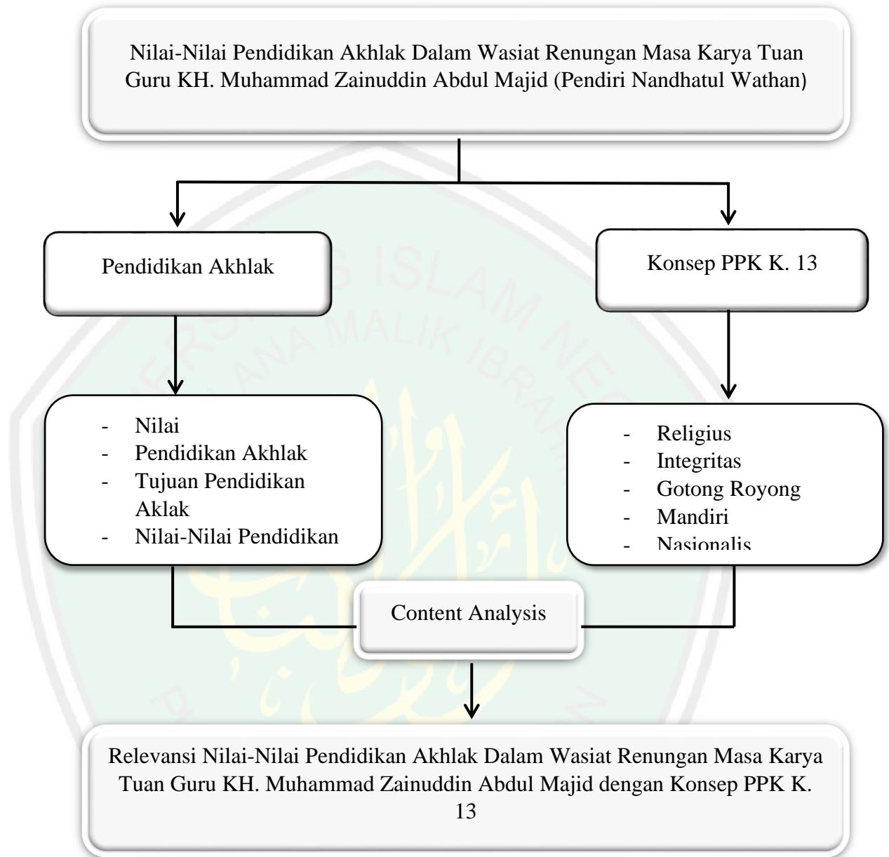
Gambar 2.2 Kerangka Berfikir
