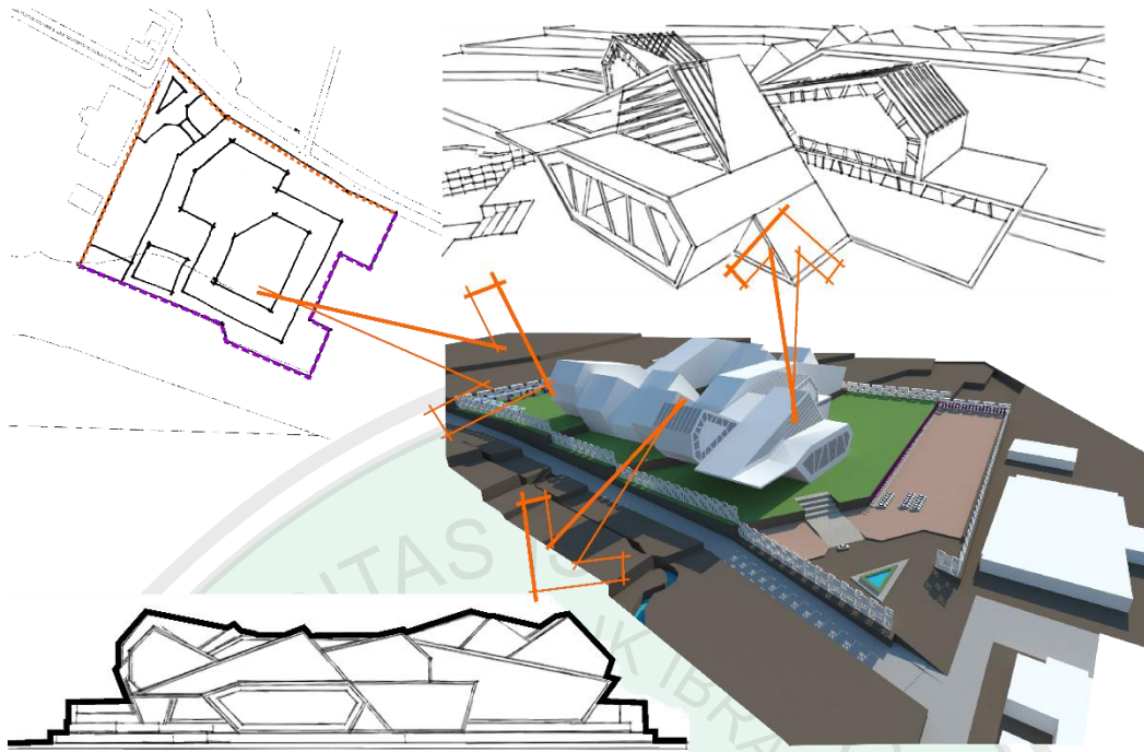
Gambar 5.1 Konsep Bentuk
