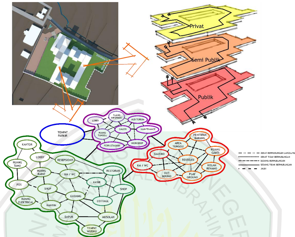
Gambar 5.3 Konsep Ruang
