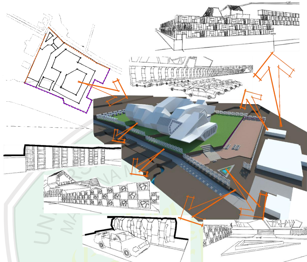
Gambar 5.2 Konsep Tapak
