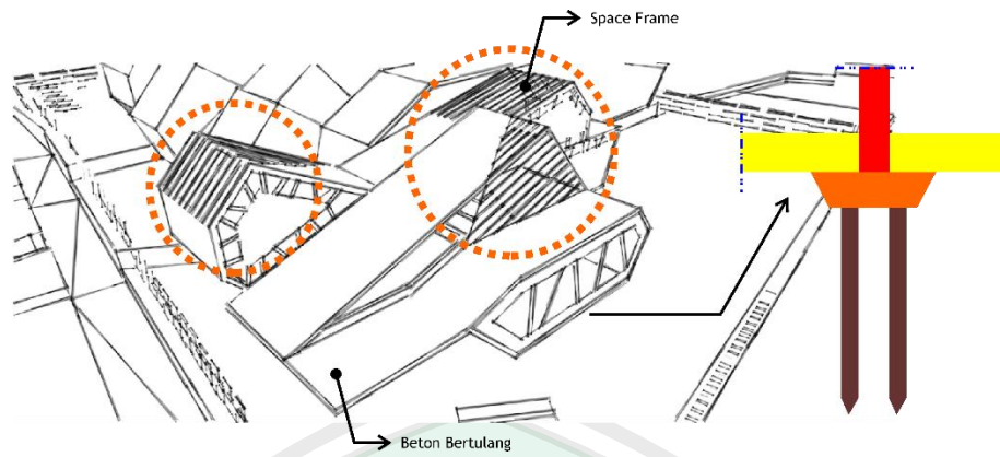
Gambar 5.4 Konsep Material
