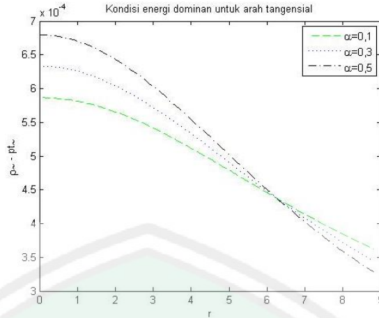
Gambar 4.10 Kondisi Energi Dominan untuk Arah Tangensial
