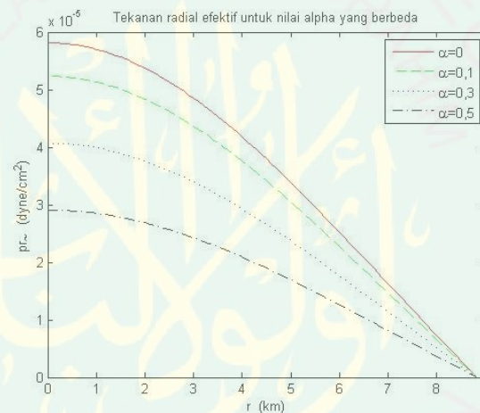
Gambar 4.6 Tekanan Radial Efektif untuk Nilai Alpha yang Berbeda
