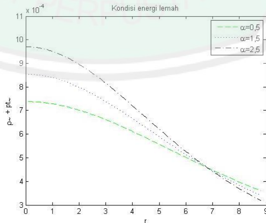
Gambar 4.13 Kondisi Energi Lemah
