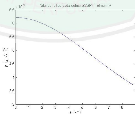
Gambar 4.1 Nilai Densitas pada Solusi SSSPF Tolman IV
