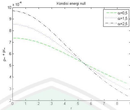
Gambar 4.12 Kondisi Energi Null
