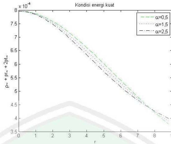
Gambar 4.11 Kondisi Energi Kuat
