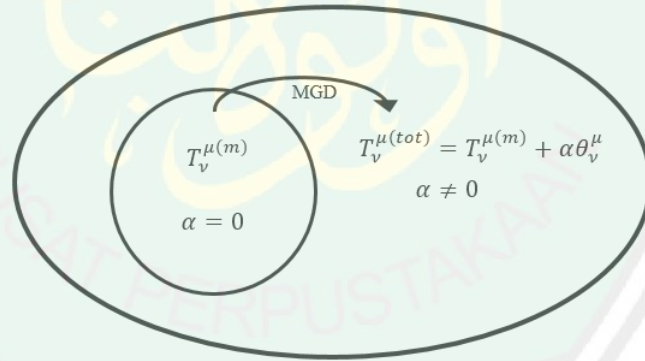
Gambar 4.4 Solusi Fluida Sempurna Apapun Secara Konsisten Diperluas ke Domain Anisotropik Melalui Metode MGD-Decoupling
