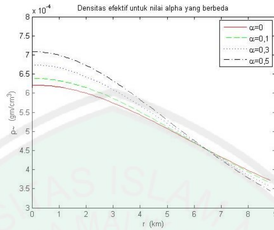
Gambar 4.5 Densitas Efektif untuk Nilai Alpha yang Berbeda
