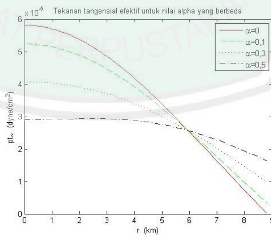
Gambar 4.7 Tekanan Tangensial Efektif untuk Nilai Alpha yang Berbeda
