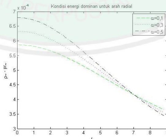
Gambar 4.9 Kondisi Energi Dominan untuk Arah Radial
