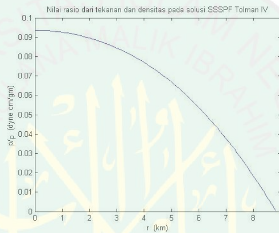
Gambar 4.3 Nilai Rasio dari Tekanan dan Densitas pada Solusi SSSPF Tolman IV
