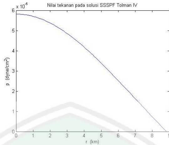
Gambar 4.2 Nilai Tekanan pada Solusi SSSPF Tolman IV
