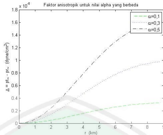
Gambar 4.8 Faktor Anisotropik untuk Nilai Alpha yang Berbeda
