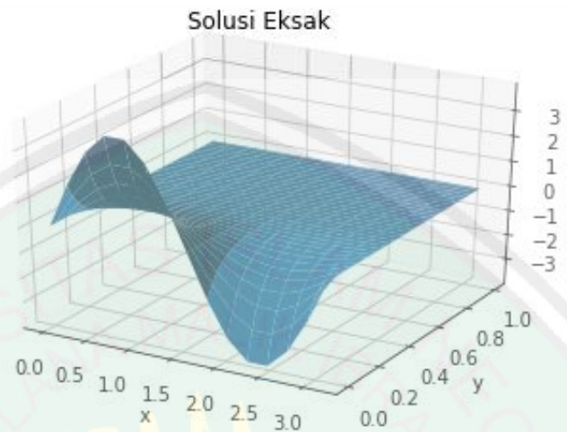
Gambar 3.12 Simulasi Ketiga Solusi Eksak Persamaan Difusi
