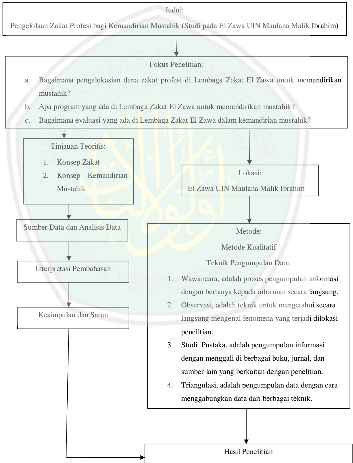
Gambar 2.1 Kerangka Berfikir
