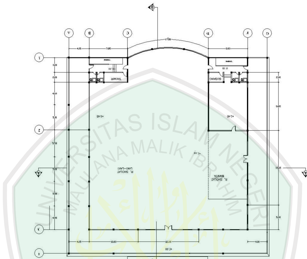
Gambar 6.20 denah Masjid Sumber: Hasil Rancangan 2013
