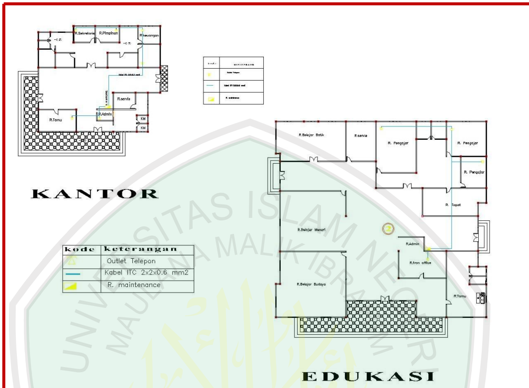
Gambar 6.34 Sistem Jaringan Telepon Sumber: Hasil Rancangan 2013
