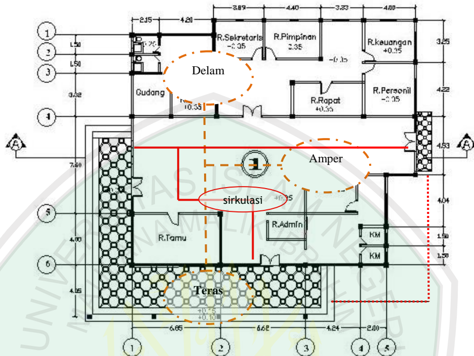
Gambar 6.18 Denah kantor Sumber: Hasil Rancangan 2013
