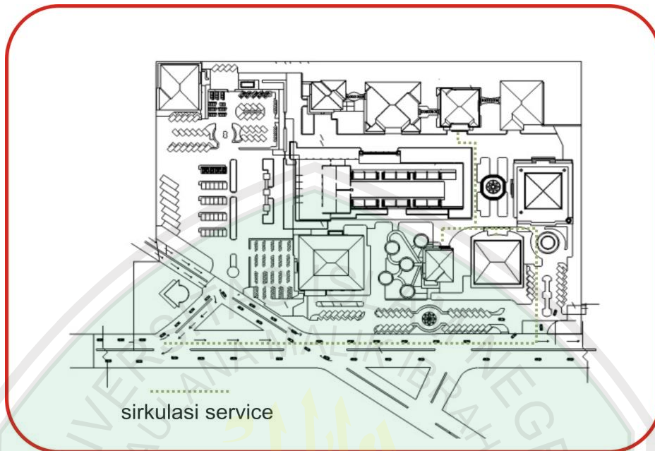
Gambar 6.4 Sirkulasi servis Sumber: Hasil Rancangan 2013
