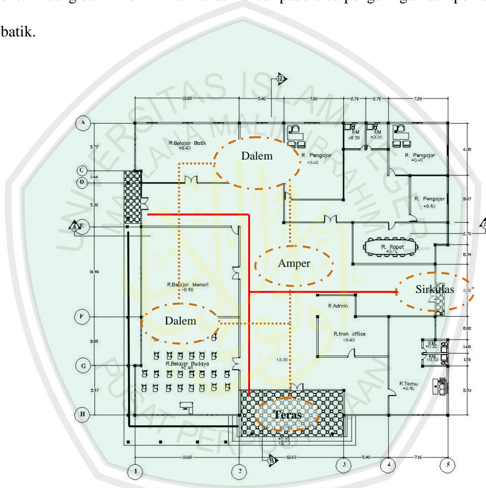
Gambar 6.6 Denah Edukasi Sumber: Hasil Rancangan 2013
