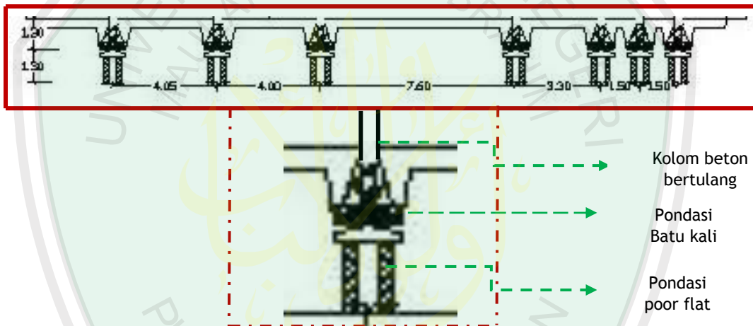
Gambar 6.29 Struktur pondasi batu kali Sumber: Hasil Rancangan 2013
