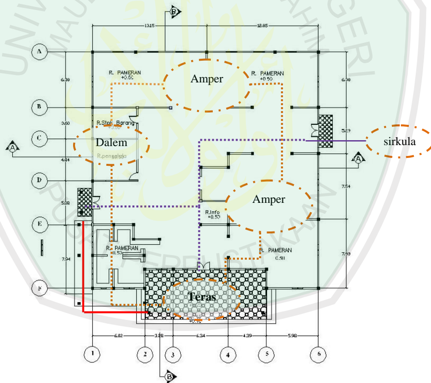
Gambar 6.8 Denah pameran Sumber: Hasil Rancangan 2013
