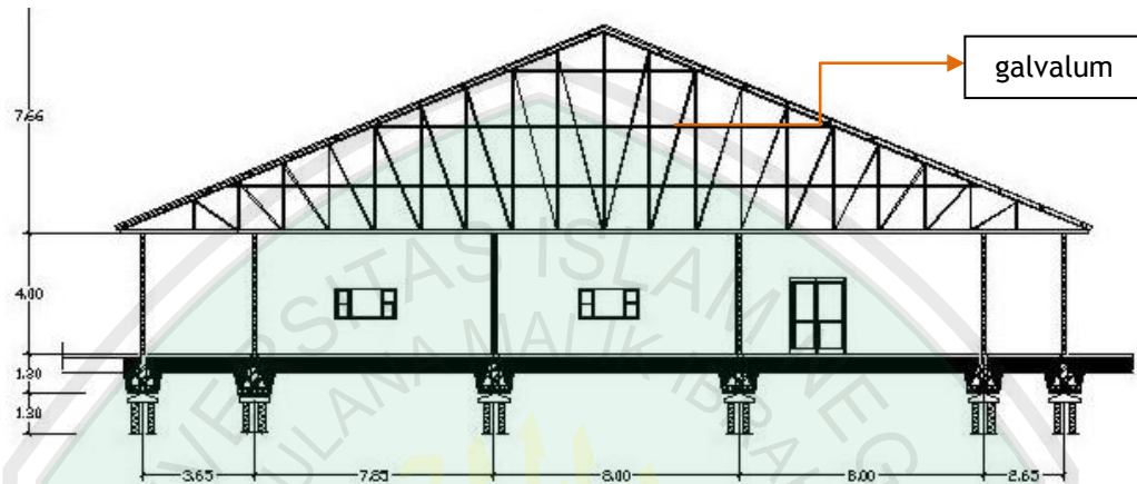
Gambar 6.30 Struktur atap galvalum Sumber: Hasil Rancangan 2013
