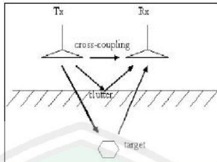
Gambar 2.16 Cross-Coupling (Telford dalam Ayik, 2009)
