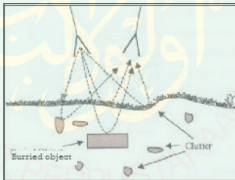
Gambar 2.15 Late Time Ringing (Telford dalam Ayik, 2009)
