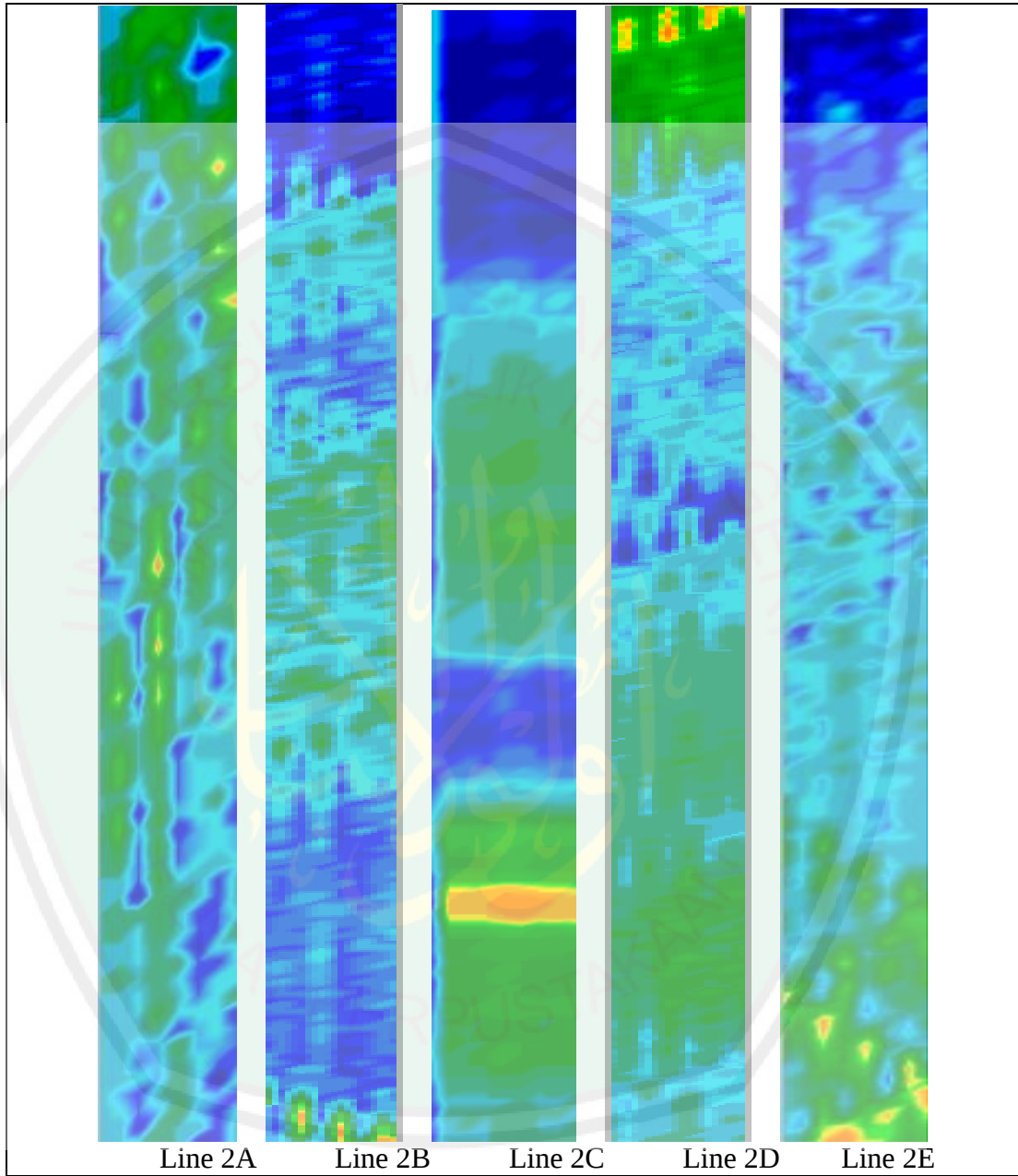
Gambar 2 Penampang Horizontal Line 2 (dari atas ke bawah : line 2A sampai line 2E)
