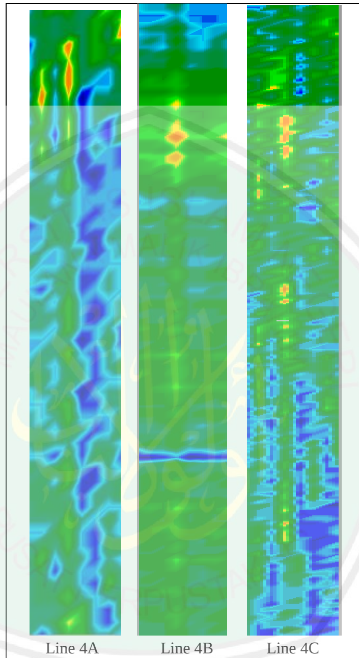
Gambar 4 Penampang Horizontal Line 4 (dari atas ke bawah : line 4A sampai line 4C)
