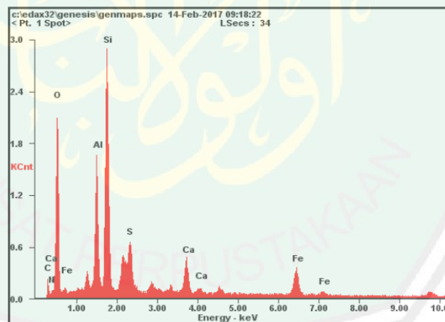
Gambar 4.3 Grafik Unsur pada Batubara Titik Kedua
