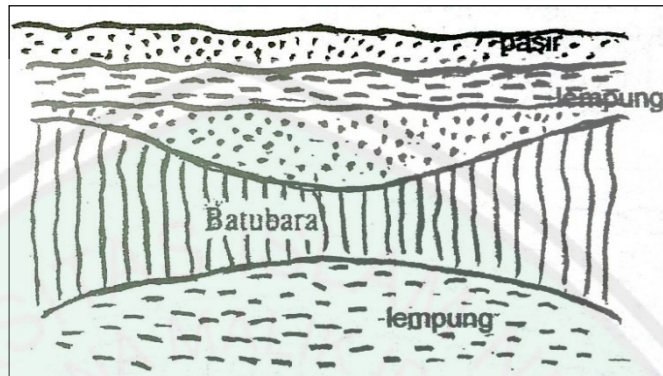
Gambar 2.6 Perlapisan Batubara Bentuk Pinch (Sumber: Sukandarrumidi, 2006)
