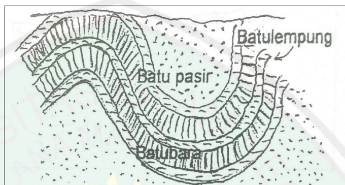
Gambar 2.10 Perlapisan Batubara Berbentuk Fold (Sumber: Sukandarrumidi, 2006)
