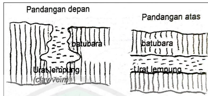
Gambar 2.7 Perlapisan Batubara Bentuk Clay Vein (Sumber: Sukandarrumidi, 2006)
