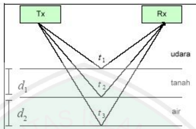
Gambar 2.14 Ketebalan Beberapa Medium dalam Tanah (Ayik, 2009)
