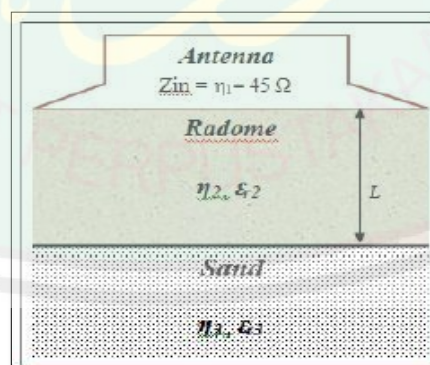
Gambar 2.17 Jarak Antena dengan Tanah (Telford dalam Ayik, 2009)
