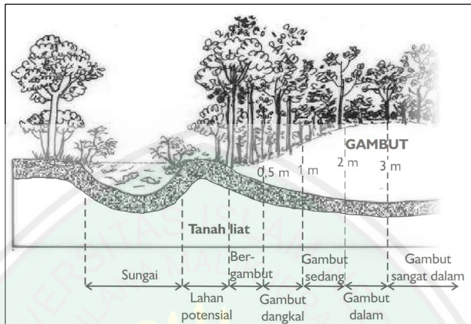
Gambar 2.3 Urutan tipe rawa gambut yang berkembang pada lingkungan Lacustrine (Taylor G.H. dkk, 1998)
