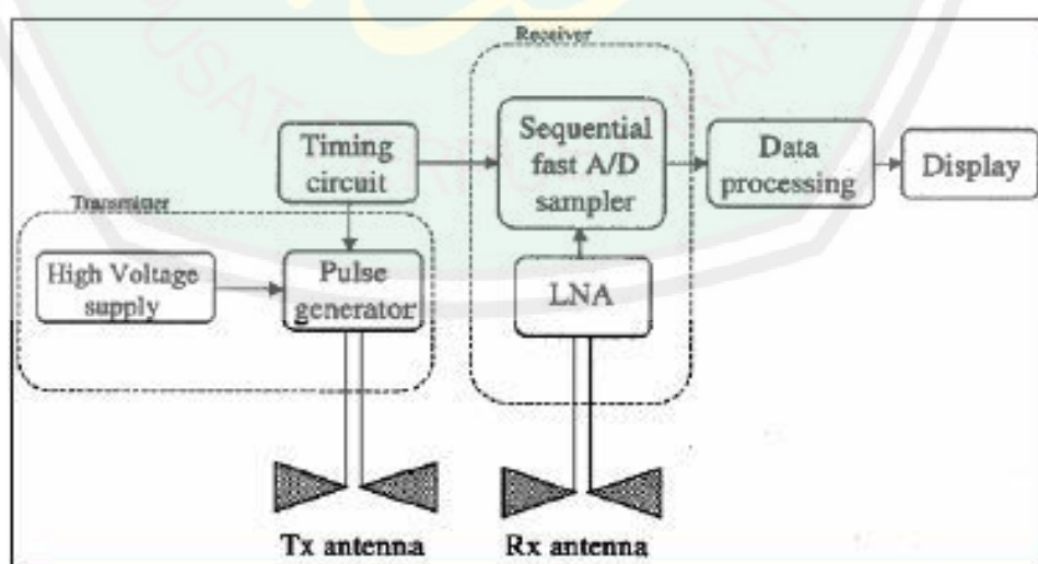
Gambar 2.13 Sistem Kerja GPR (Ligthart dalam Ayik, 2009)
