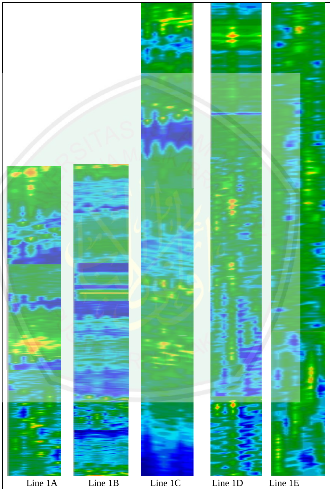
Gambar 1 Penampang Horizontal Line 1 (dari atas ke bawah : line 1A sampai line 1E)
